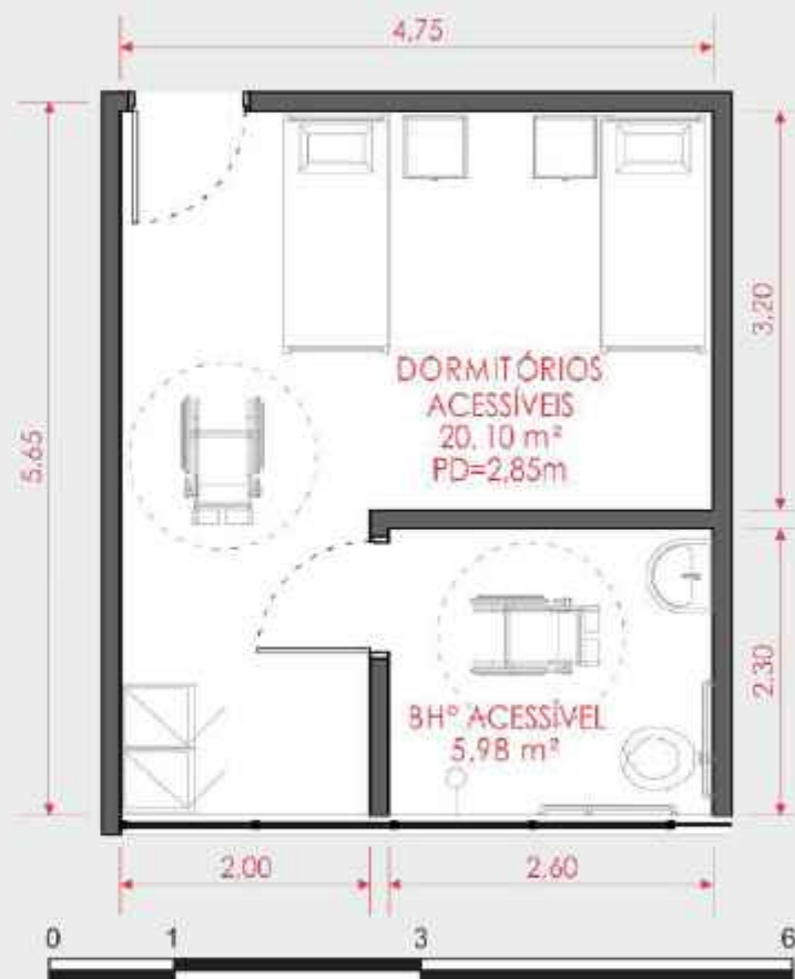
02 PLANTA BAIXA DORMITÓRIOS ACESSÍVEIS
