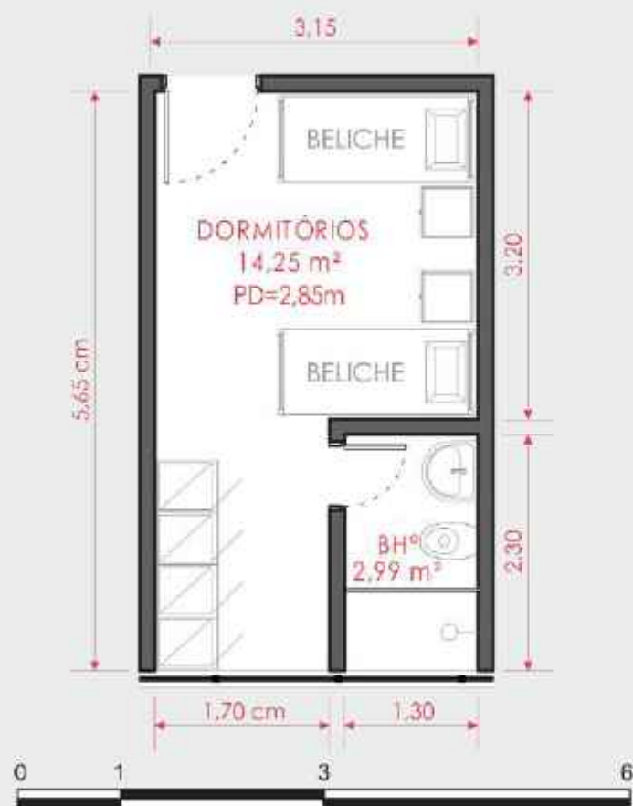
01 PLANTA BAIXA DORMITÓRIOS COMUNS
