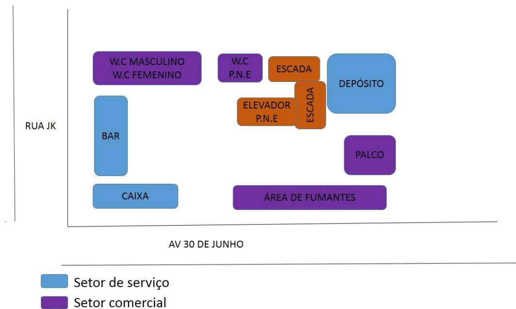
Figura 45: Fluxograma
