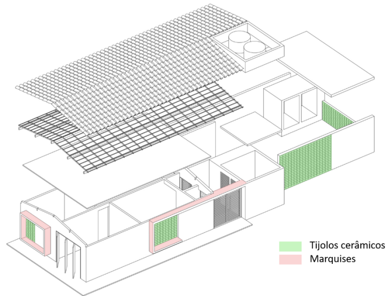
Figura 20: Elementos arquitetônicos da volumetria
