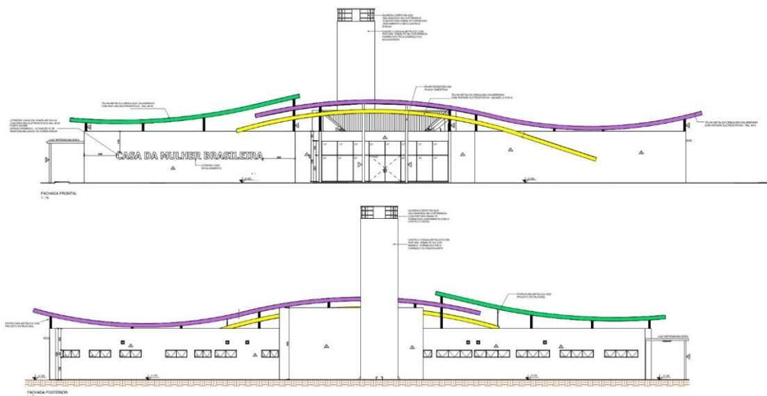
Figura 16: Fachada frontal e posterior
