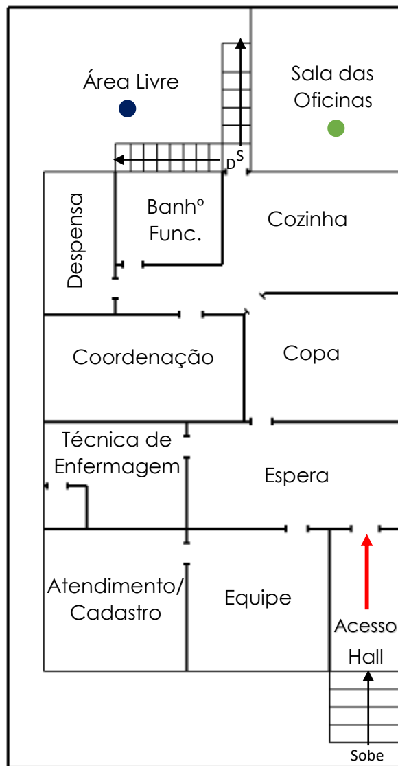
Figura 52 – Croqui Centro POP Ubá – 1º pavimento. Fonte: Autoria Própria
