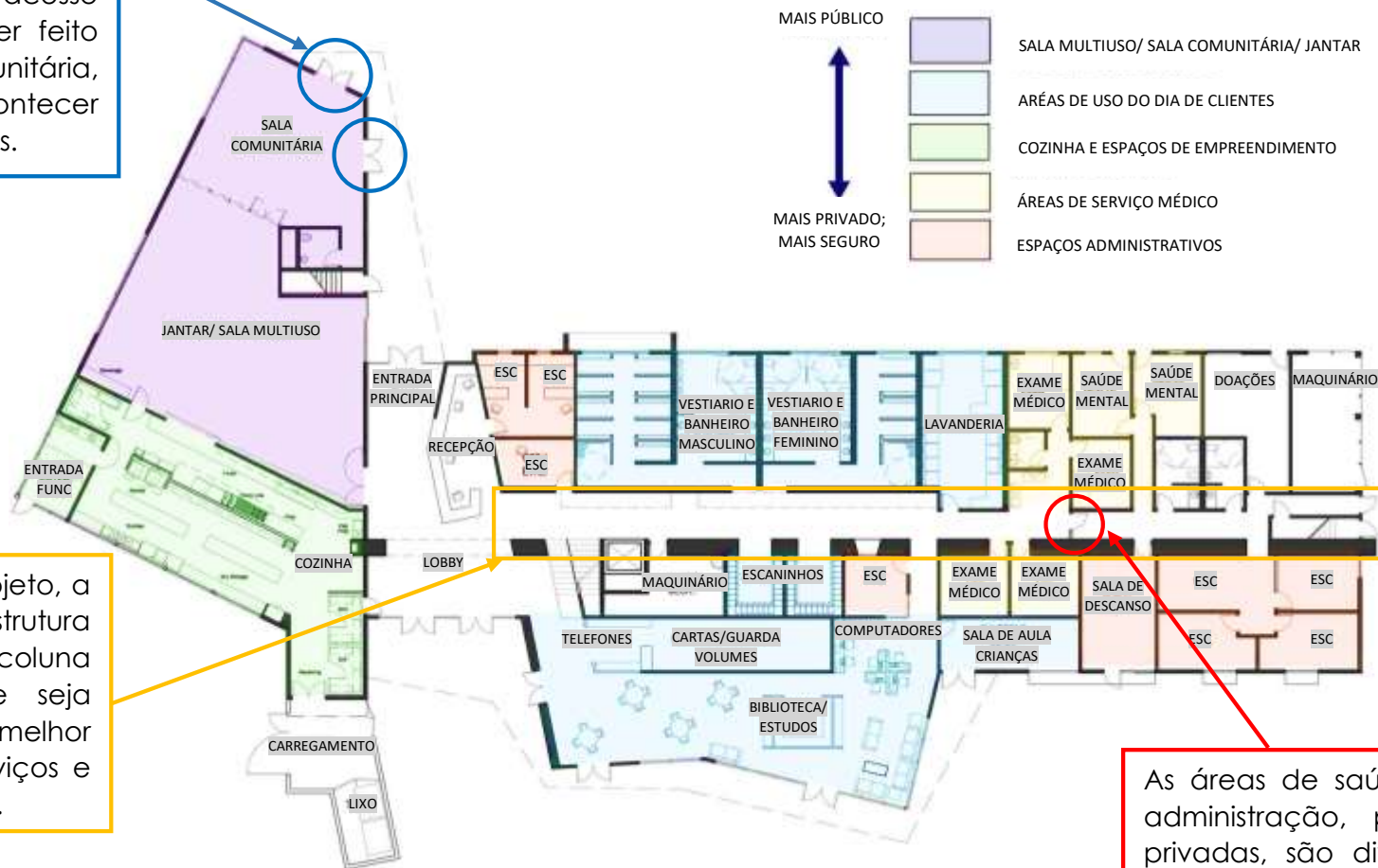
Figura 62 - Planta baixa térreo setorizada Fonte: ArchDaily editada pelo autor
