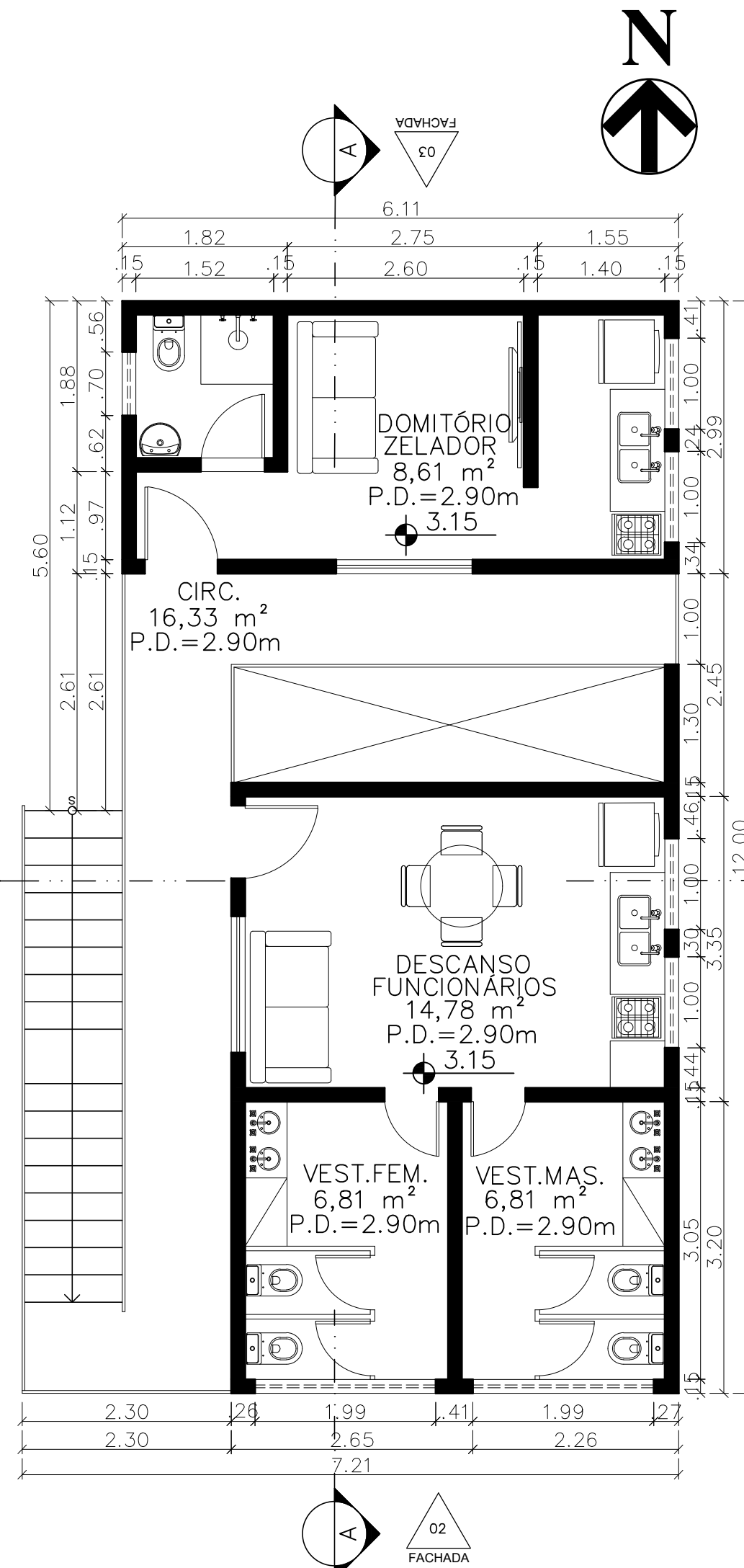
01 PLANTA BAIXA 2º PAV APOIO ABRIGO ESC.1/100
