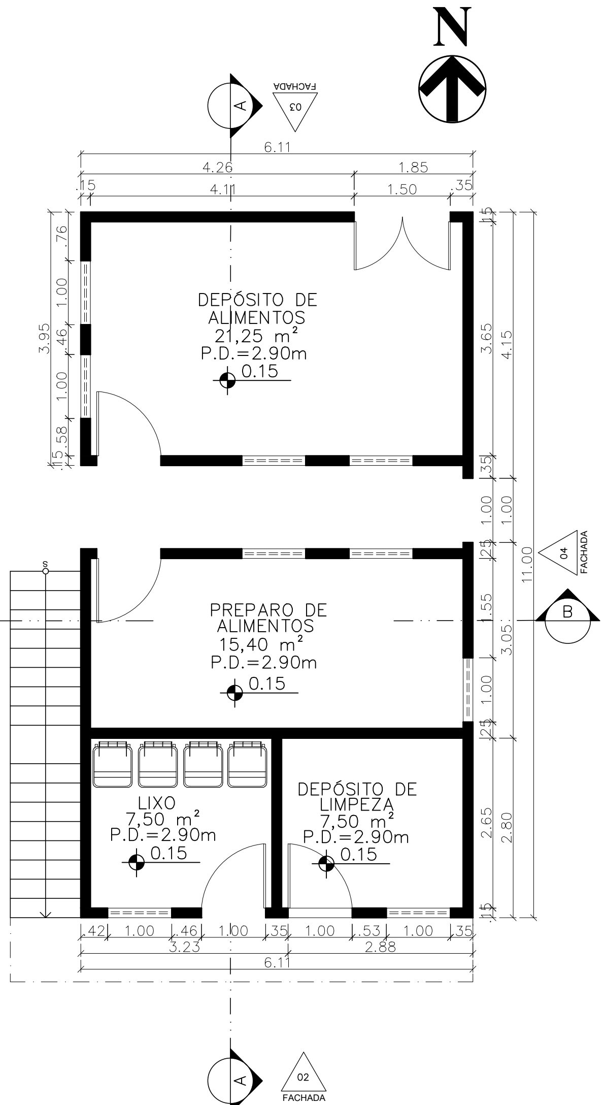
01 PLANTA BAIXA TÉRREO APOIO ABRIGO ESC.1/100
