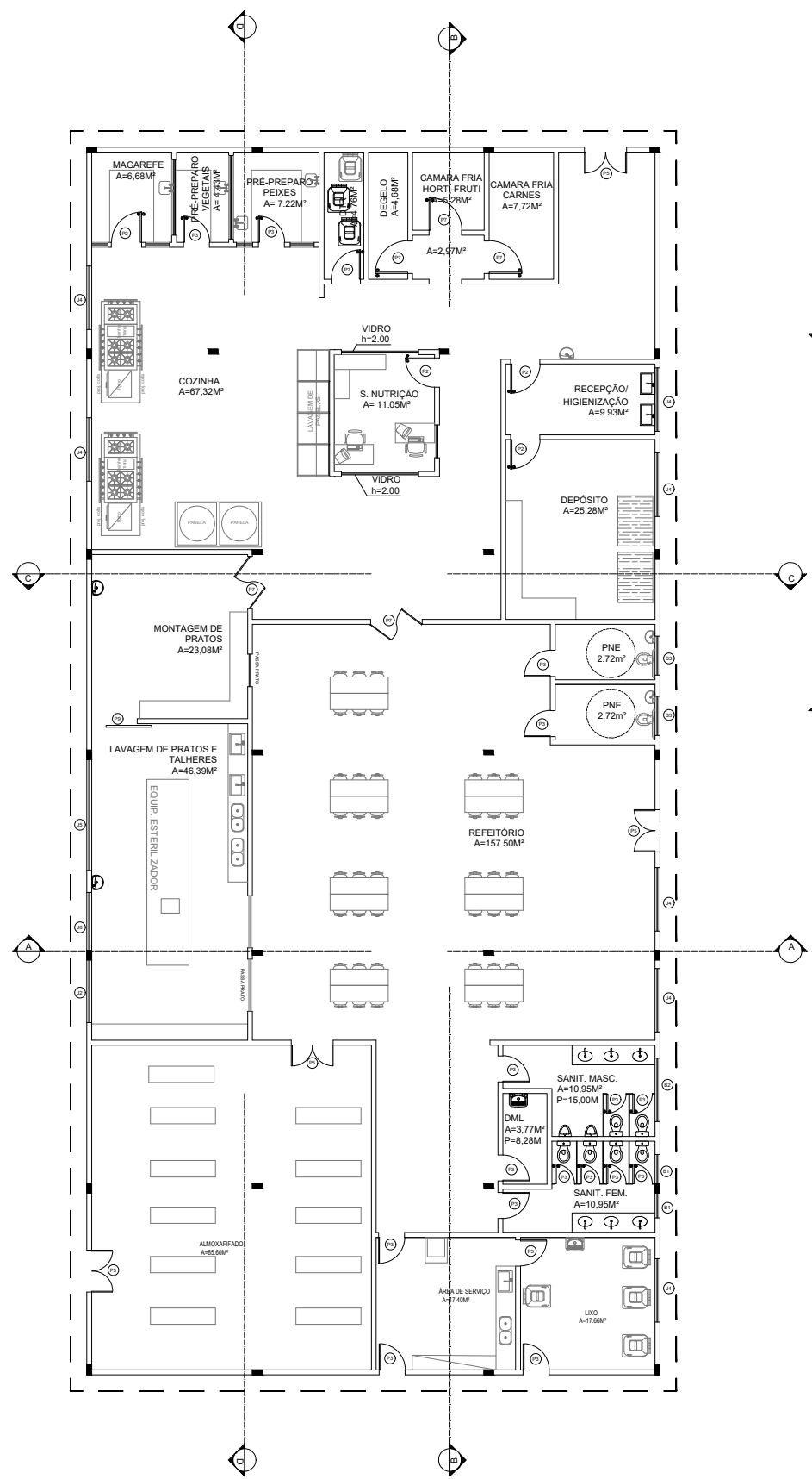
3 PLANTA BAIXA - BLOCO SERVIÇO ESC: 1/100
