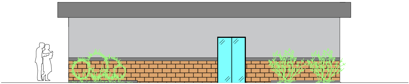
1 FACHADA FRONTAL - BLOCO ADM ESC: 1/100
