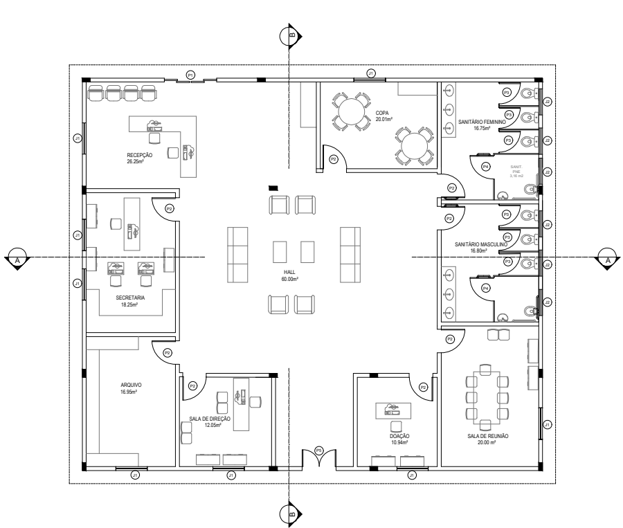
1 PLANTA BAIXA - BLOCO ADM ESC: 1/200
