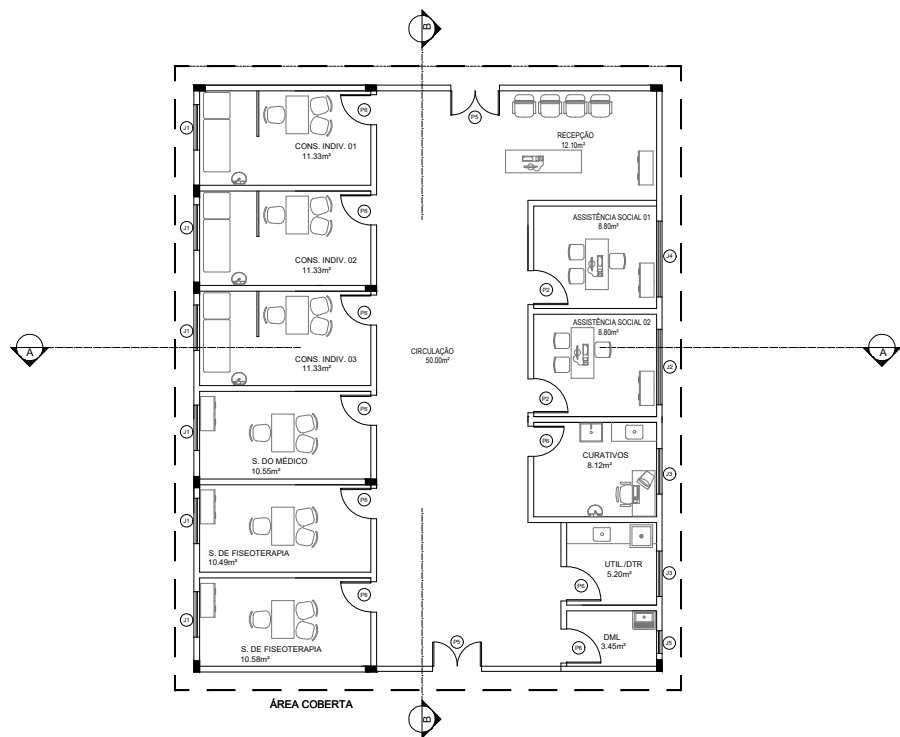
2 PALNTA BAIXA - BLOCO SERVIÇO ESC: 1/100
