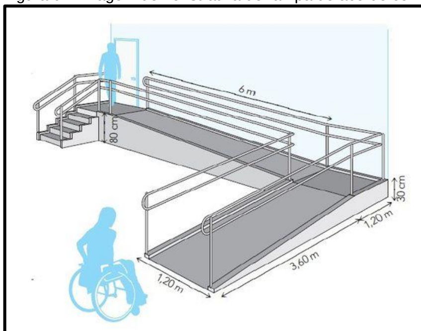
Figura 02: Imagem demonstrativa de rampa de acordo com NBR 9050
