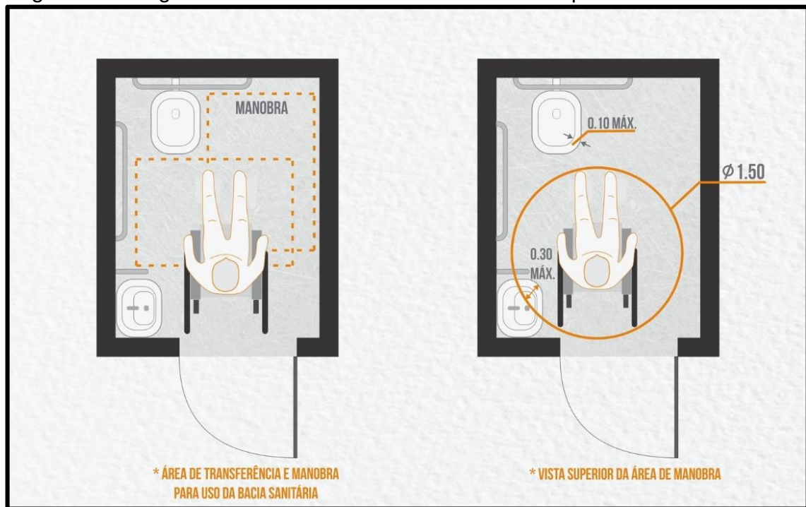
Figura 69: Imagem demonstrativa de medidas mínimas para banheiro PNE
