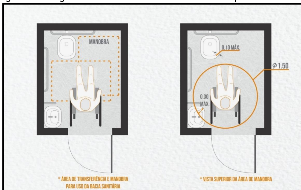
Figura 03: Imagem demonstrativa de medidas mínimas para banheiro PNE
