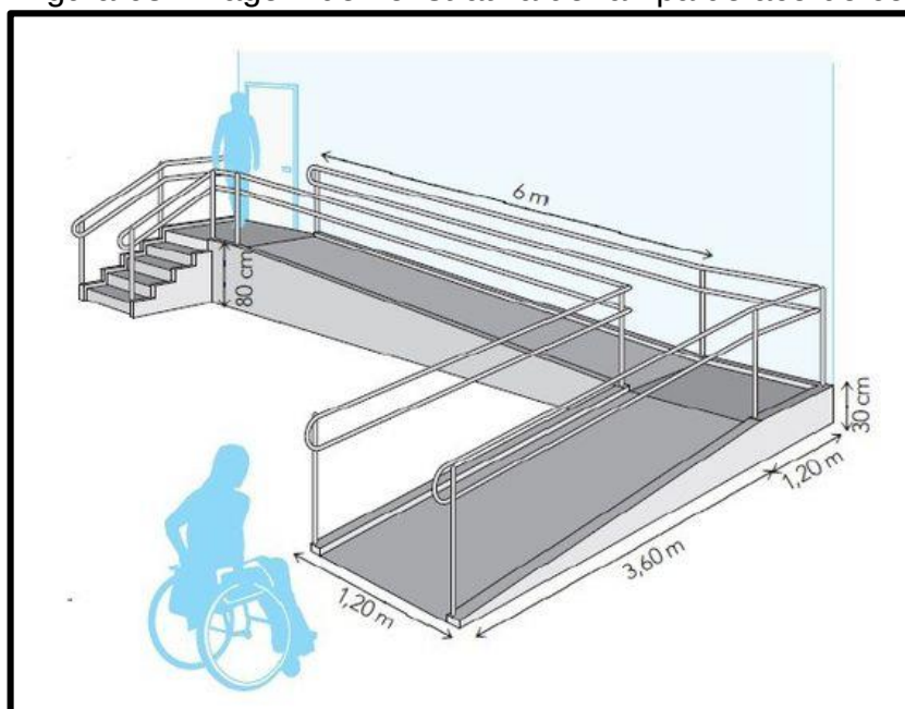
Figura 68: Imagem demonstrativa de rampa de acordo com NBR 9050
