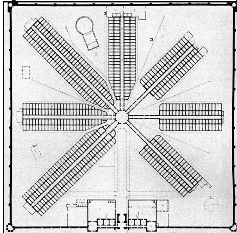
Figura 22: Desenho da Planta da Penitenciária Cherry Hill
