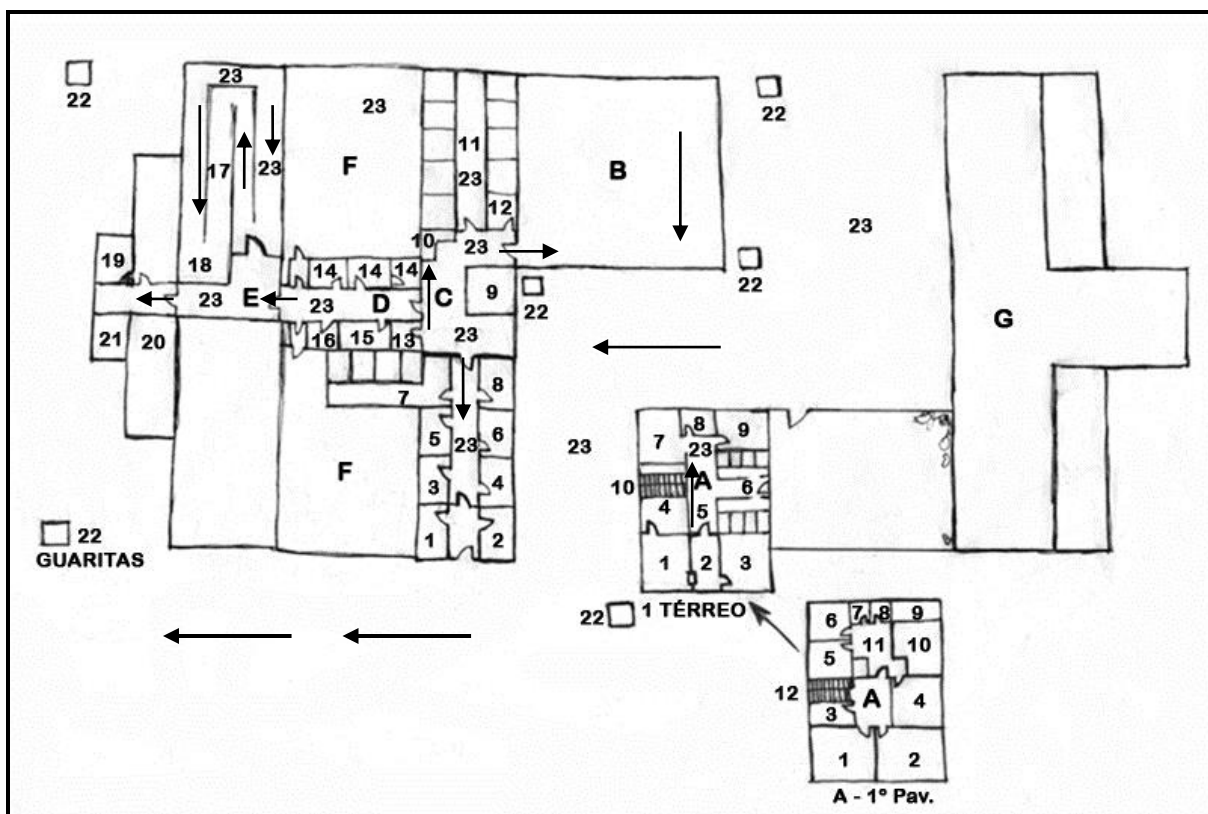
Figura 45 – Planta Casa de Custódia de Itaperuna Fonte: Autoria própria
