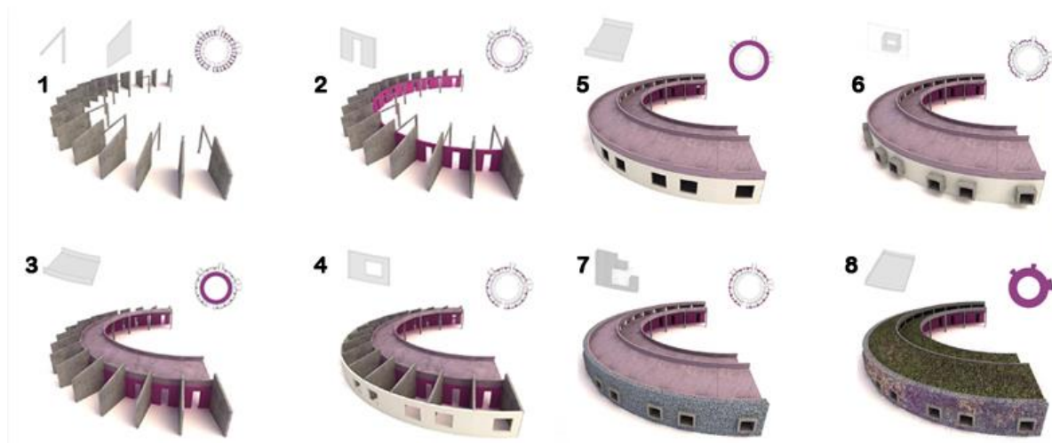
Figura 92 – Etapas da montagem passo a passo do bloco de celas
