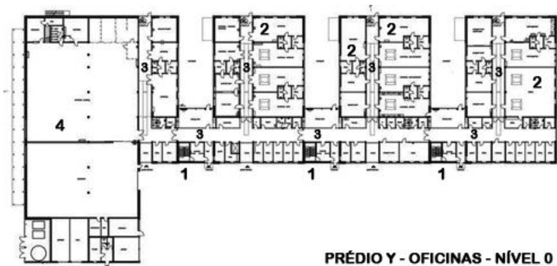
Figura 54 - Prédio Y, oficinas Fonte: OpenBuildings (2015)
