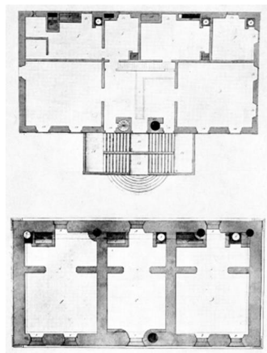
Figura 10 - Plantas do pavimento térreo e do sobrado da antiga Casa de Câmara e Cadeia de Mariana-MG, 1830 Fonte: Oliveira (2007)
