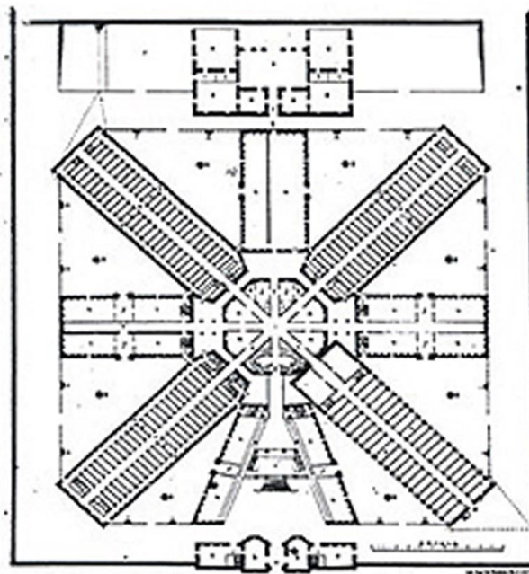
Figura 11 – Planta da Casa de Correção da Corte do Rio de Janeiro 1834 Fonte: Pessoa (2013)
