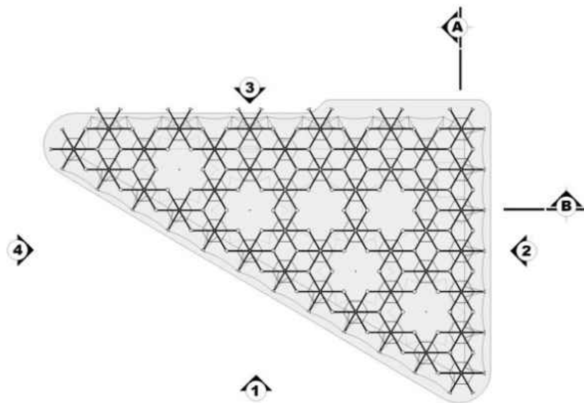
PLANTA DE ESTRUTURA
