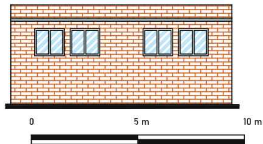
FACHADA LATERAL
