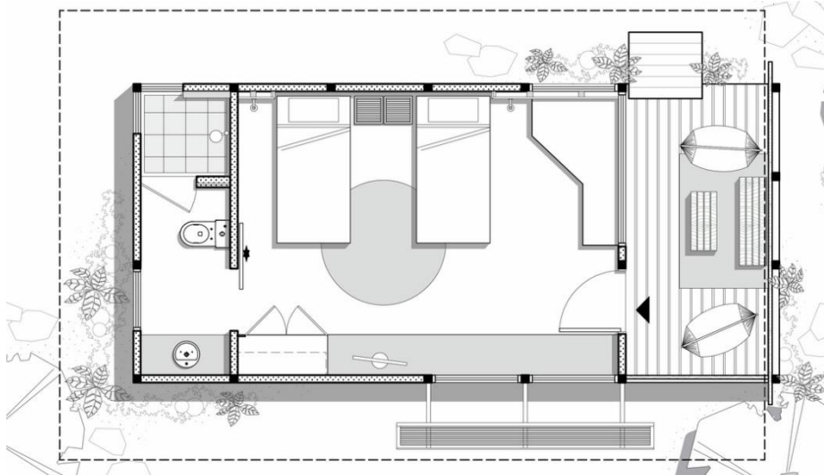
Figura 17 - Layout dos 'bungalows' do Hotel Rio Perdido.
