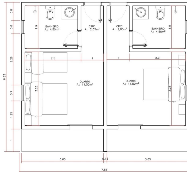
Figura 8 - Croqui do layout do item 4 e 5.
