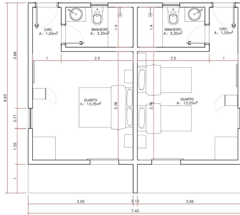
Figura 7 - Croqui do layout dos itens 1 e 3.
