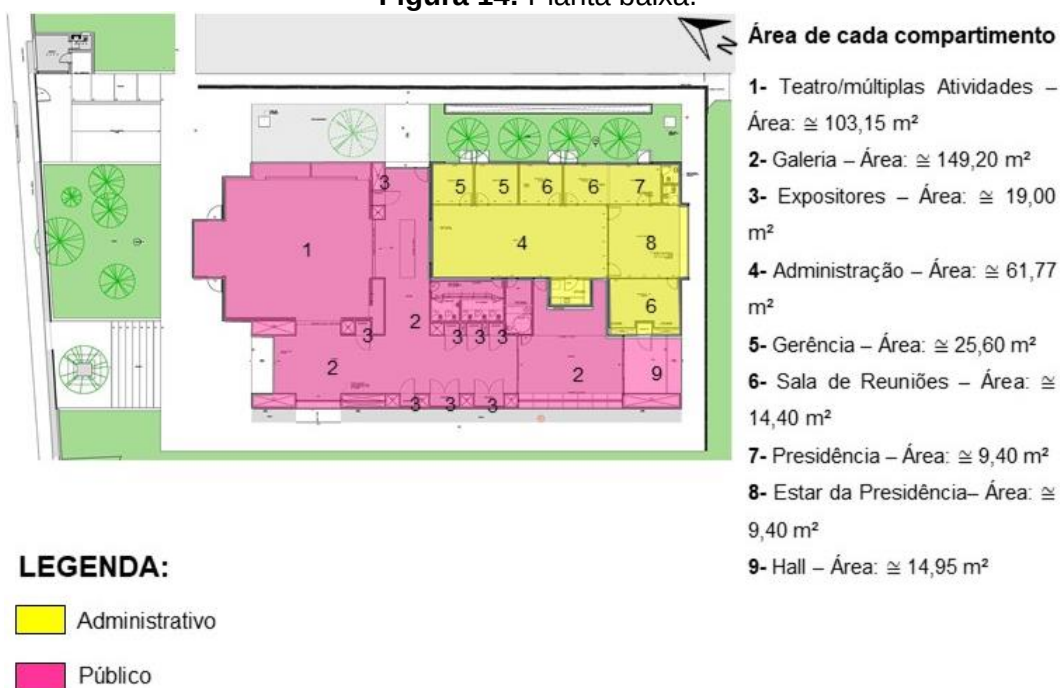
Figura 14: Planta baixa.
