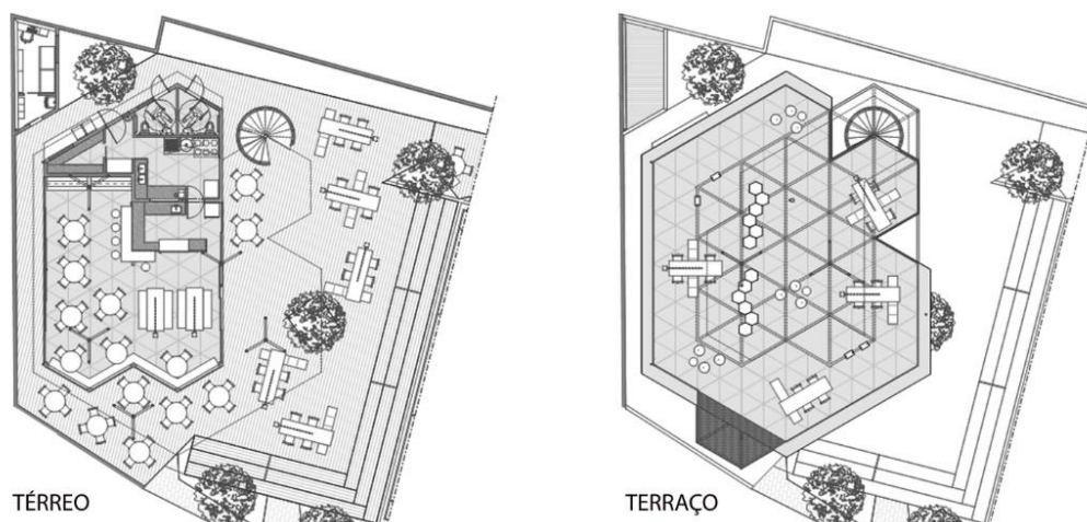
Figura 73: Planta baixa do térreo e terraço.
