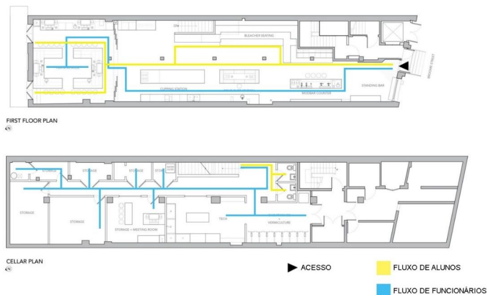
Figura 35: Fluxos e acessos do primeiro e segundo pavimento.
