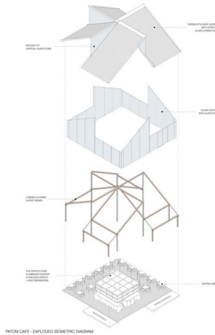
Figura 50: Esquema da estrutura.
