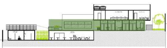
CORTE A
