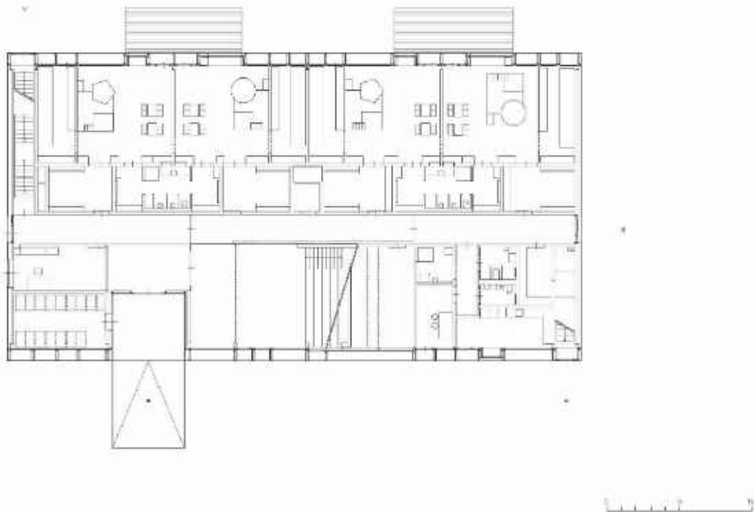
Figura 8: Planta baixa da creche.
