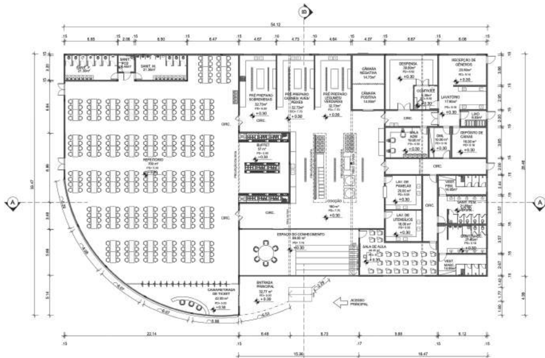
1 PLANTA BAIXA ESCALA INDICADA
