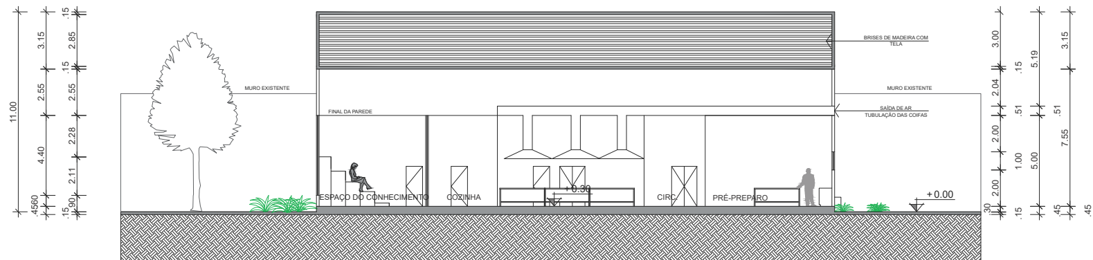
2 CORTE TRANSVERSAL - BB ESCALA INDICADA
