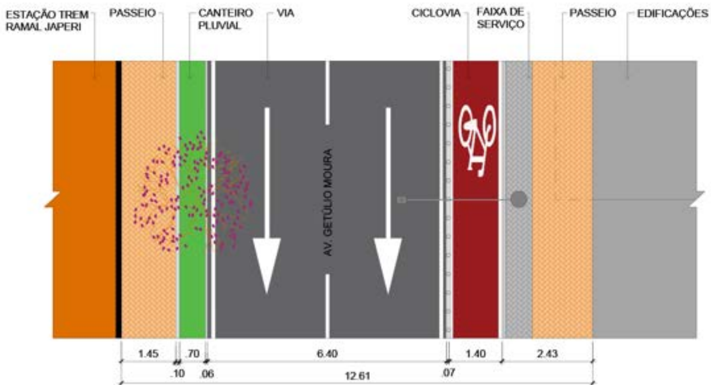
PLANTA BAIXA TECHO DA AV. GETULIO MOURA Esc.1:100
