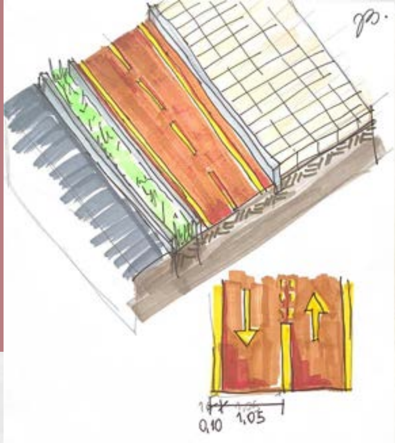
Figura 65: Croqui ciclovia bidirecional Croqui elaborado pela autora
